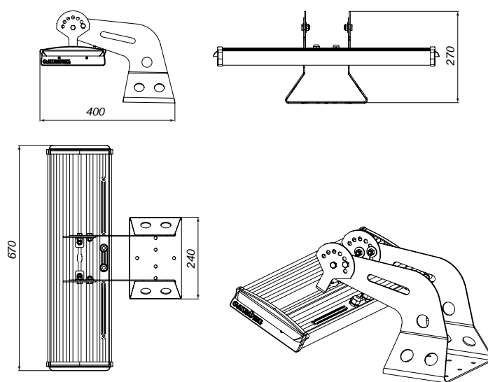
Общий вид 4-модульного светильника
