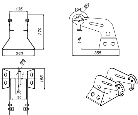
Кронштейн универсальный (габаритные размеры)
