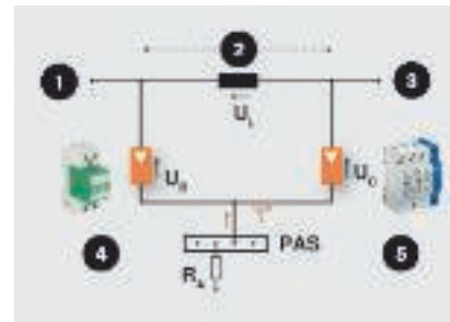
1= сетевое питание, 2 = провод, 3 = потребитель, 4 = напряжение срабатывания 2 кВ, например, MC 50-B VDE; 5 = напряжение срабатывания 1,4 кВ, например, V20 C
