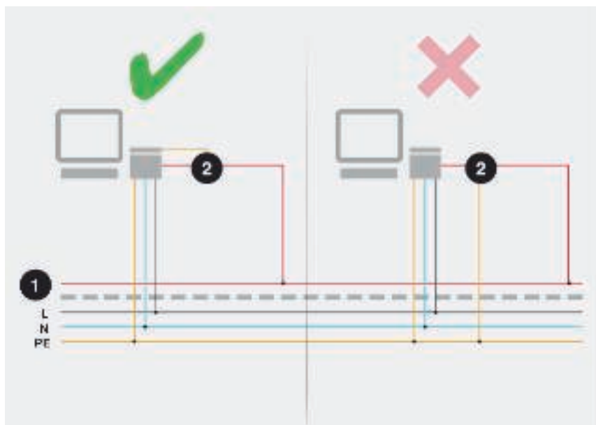
Указания по монтажу: 1 = сеть ISDN, 2 = защитное устройство
