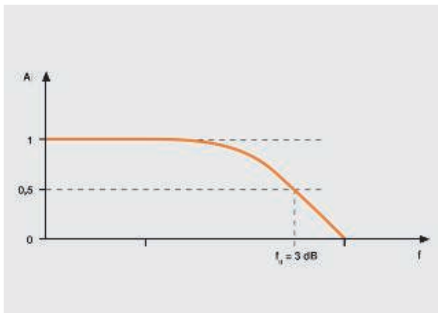
Демпфирование в диаграмме Бode
