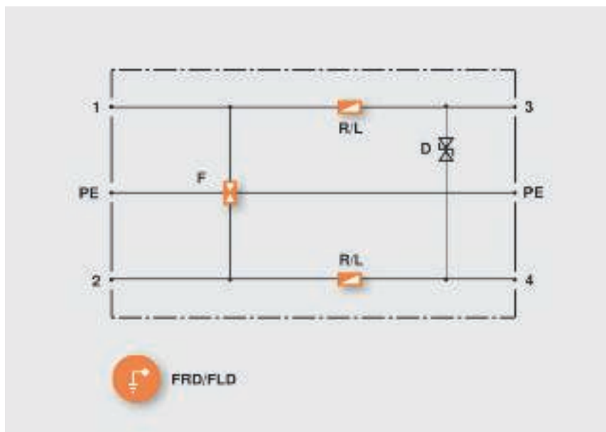
Схема молниезащитного барьера FRD/FLD
