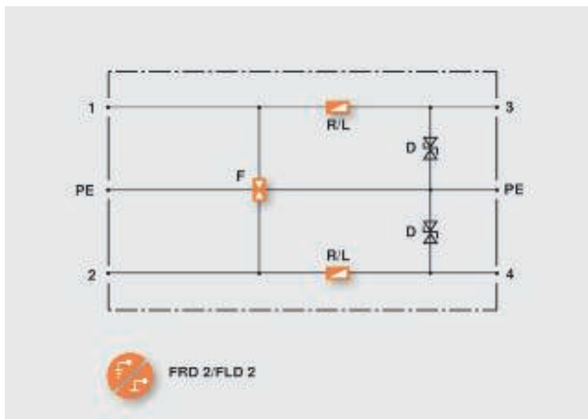
Схема молниезащитного барьера FRD2/FLD2
