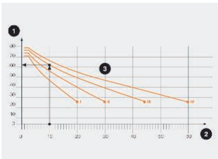
1 = защитный угол \alpha^\circ , 2 = высота уступа ( h ) в м, 3 = классы молниезащиты I/II/III/IV
