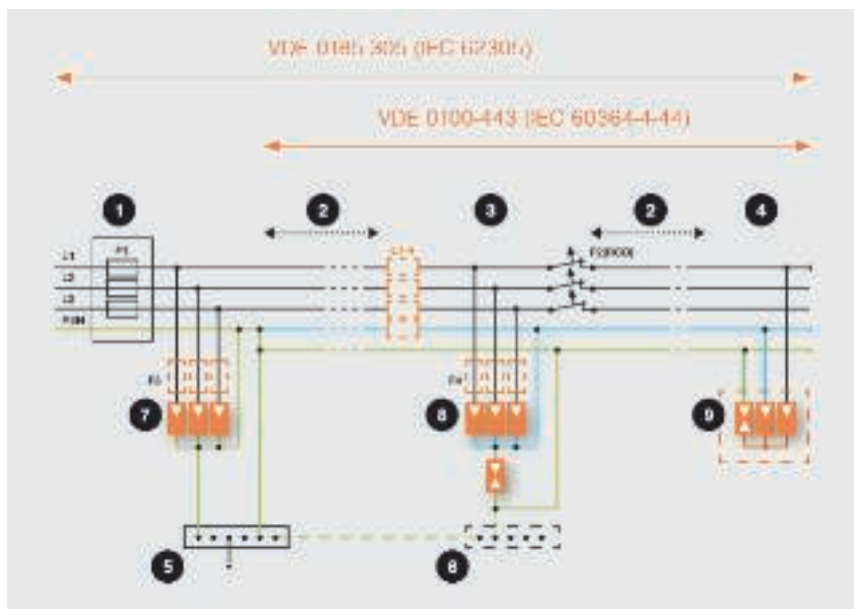
1 = главное распределительное устройство, 2 = длина провода, 3 = распределитель электрической цепи, например, вторичный распределитель, 4 = высокочувствительное устройство защиты сети, 5 = главная шина уравнивания потенциалов, 6 = локальная шина уравнивания потенциалов, 7 = разрядник типа 1, 8 = разрядник типа 2, 9 = разрядник типа 3
