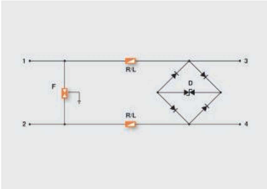
Переключение базовой защиты в измерительной цепи
