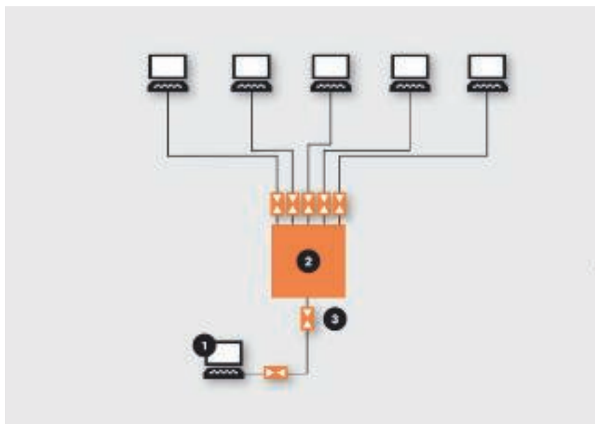
1 = сервер, 2 = коммутатор/концентратор, 3 = устройства защиты от перенапряжений
