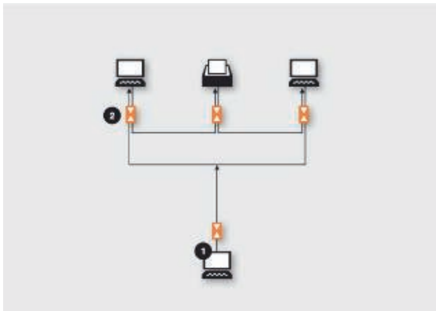
Количество жил зависит от типа сети. 1 = сервер, 2 = устройства защиты от перенапряжений
