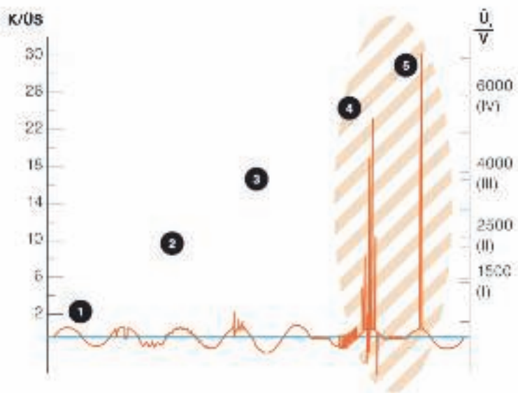
Переходные перенапряжения: 1 = резкие увеличения напряжения/краткие перерывы, 2 = высокие гармоники из-за медленных и быстрых изменений напряжений, 3 = временные повышения напряжения, 4 = коммутационные перенапряжения, 5 = перенапряжения из-за молнии, на сечка = применение устройств защиты от перенапряжений
