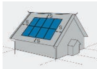
Рисунок 2: разделительный интервал ( s ) между системой молниезащиты и фотогальванической установкой
