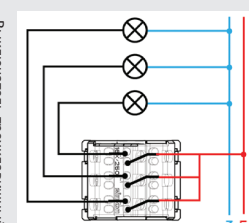
Выключатель трехклавишный
