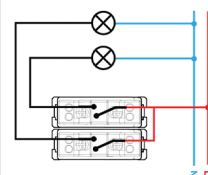
Двойной выключатель
