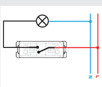
Выключатель однополюсный
