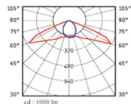
СДКУ-М-LED54 тип КСС - Ш
