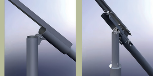
Узел складывания СТО 10,0-14,0
