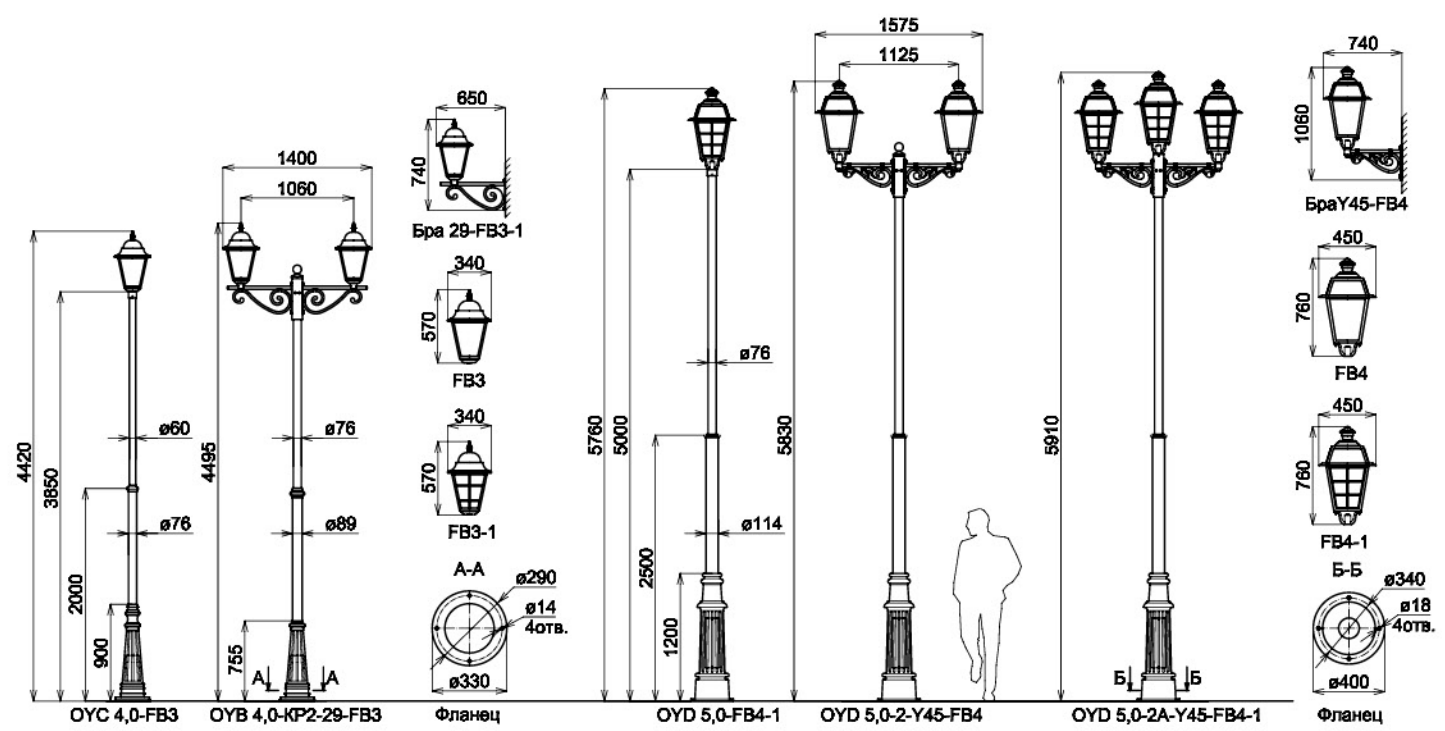
FB4-LED54 (d76) цвет ЧС 1202027350 FB4 (d76) цвет ЧС 1202023150 FB4-1 (d76) цвет ЧС 1202023160
