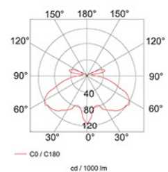
ЖТУ 06-70 с Аурис макси
