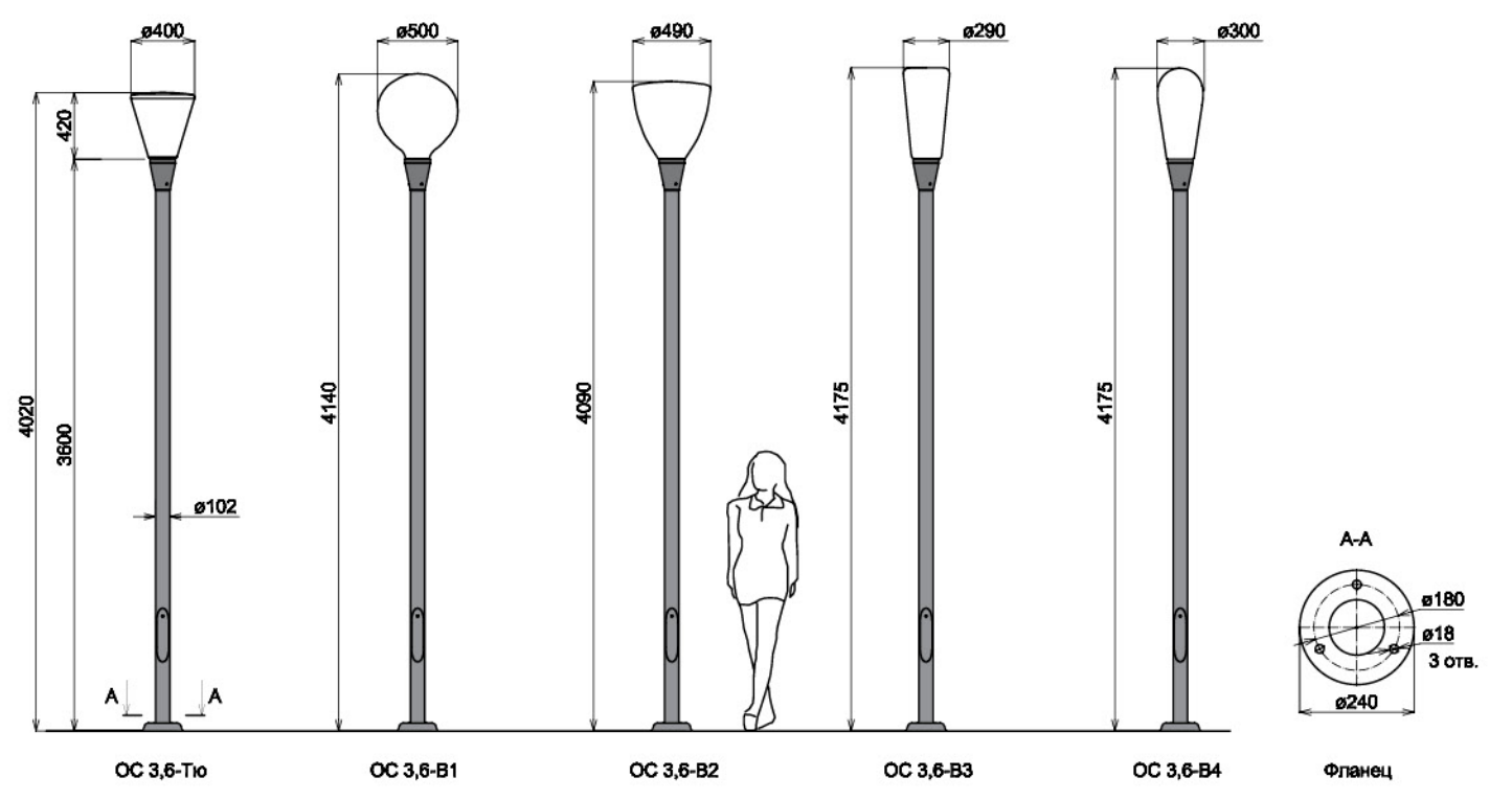
Тюльпан 734936/05 прозр. зерк. верх серебро 267005 Баллон В4 742529/45 прозр. матиров. 121267 Тюльпан В2 735174/05 прозр. зерк. верх серебро 268711 Конус В3 742528/45 прозр. матир. 121263 Шар В1 742530/45 прозр. 120914
